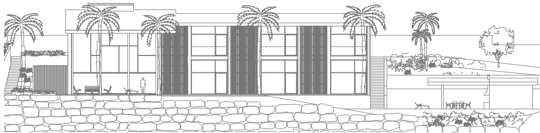
Alzado Oeste/West Elevation
